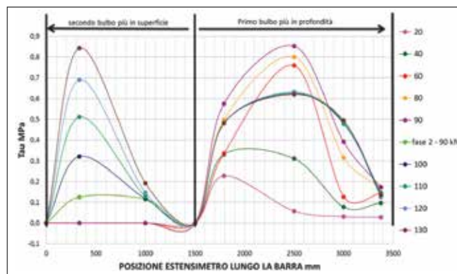
distribuzione \tau lungo l'ancoraggio al termine di ciascun ciclo di carico
