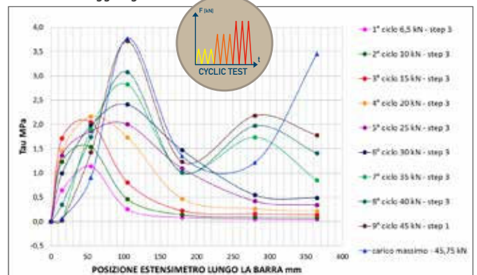
distribuzione \tau lungo l'ancoraggio (valori riferiti al 3° step di ogni ciclo)
