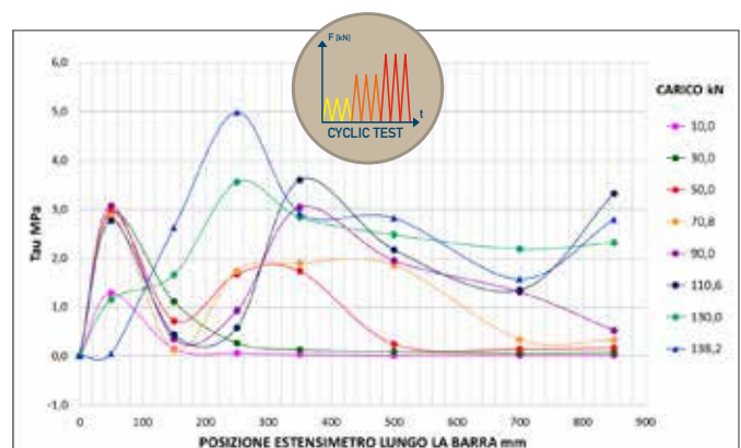
distribuzione \tau lungo l'ancoraggio
