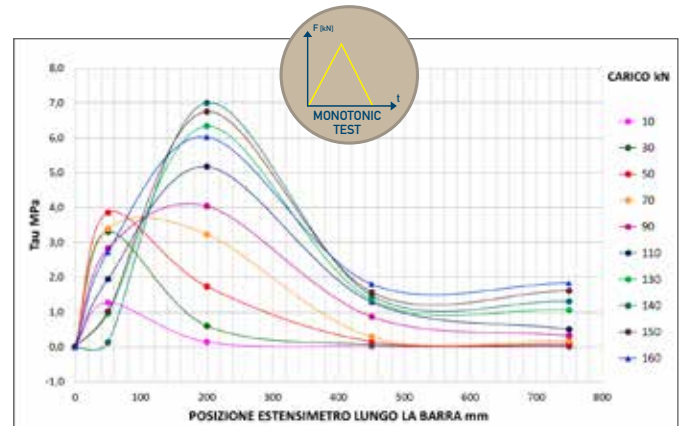
distribuzione \tau lungo l'ancoraggio ( l_{eff} = 900 mm)
