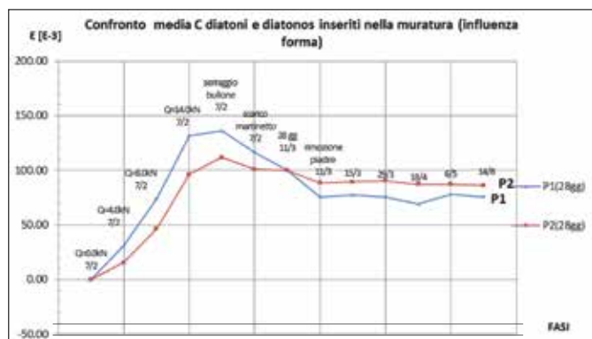
confronto tra Diatoni e Diatonos a 28 gg valori espressi in termini di deformazioni residue e misurati nella sezione centrale (C)
