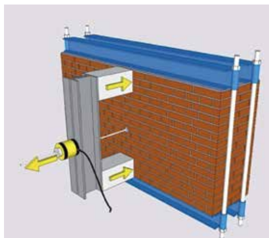
schema del banco prova e del layout generale di prova
