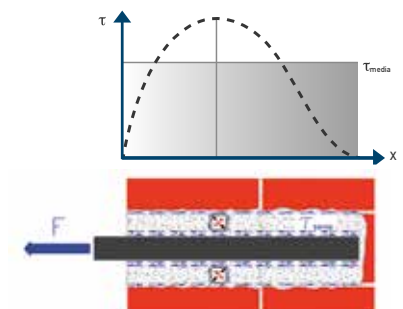
distribuzione sollecitazioni nell'ancoraggio all'interfaccia barra-malta e bulbo malta-substrato
